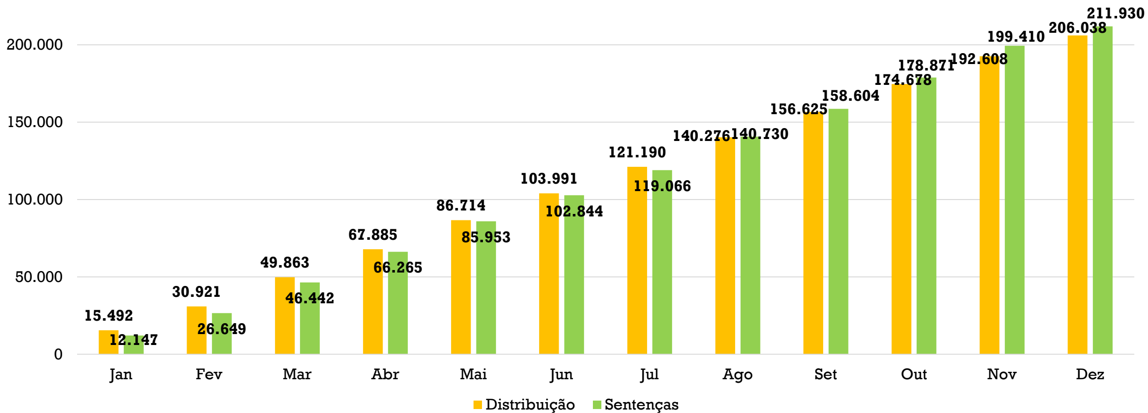
Dados acumulados
