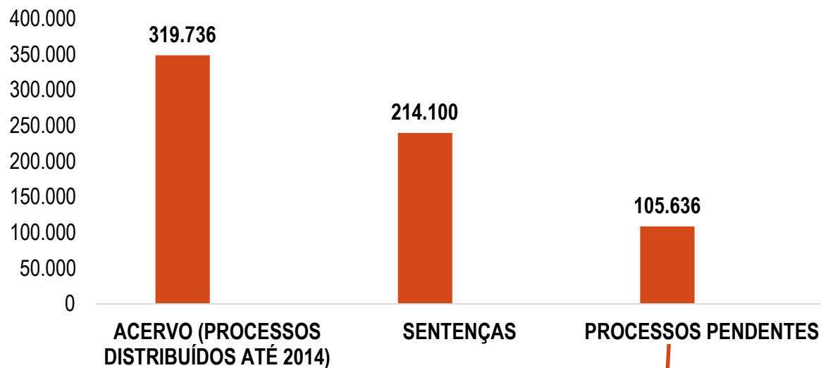
RESULTADO 2018
