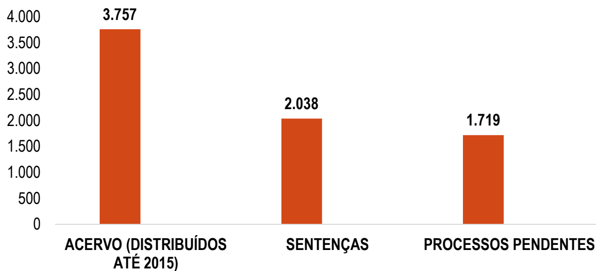
RESULTADO 2018
