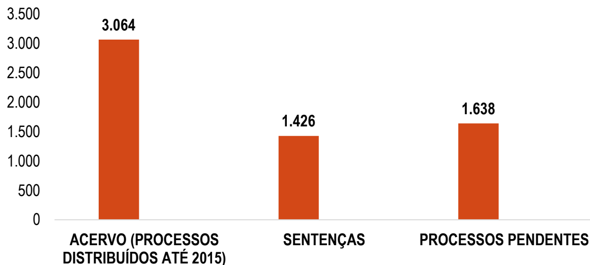
RESULTADO 2018
