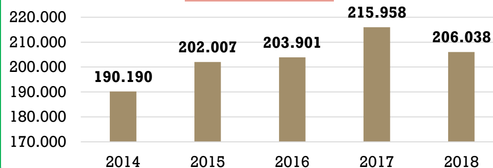
Distribuição
