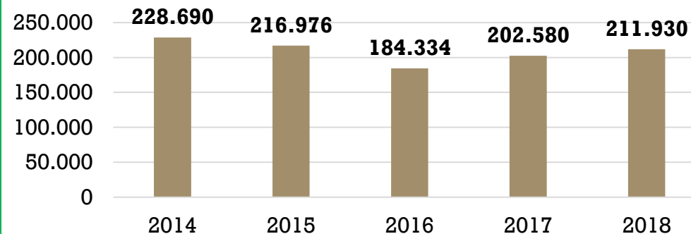
Sentenças
